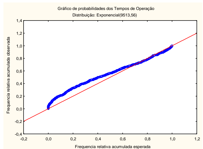
Fig. 4. Gráfico de probabilidades dos TTF dos transformadores: aderência à distribuição exponencial
