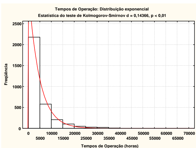
Fig. 3. Histograma dos TTF das linhas de transmissão: aderência à distribuição exponencial
